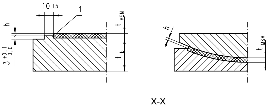
Abb. B.1 — Einzelheiten der MSM ® Kammerung und des Überstandes
