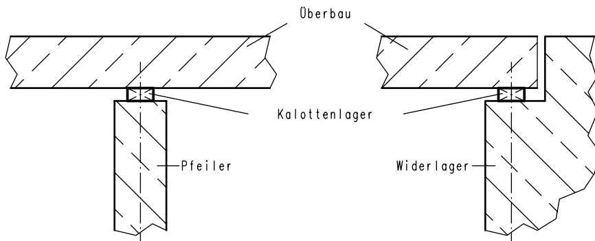
Abb. A.1 — Zusammenbau eines geführten und allseits beweglichen MSM® Kalottenlagers und vorgesehener Verwendungszweck (Beispiel)
