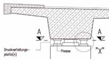
3 Pressenanordnung auf Unterbauten; Richtzeichnung Lag 6, 2009 © Bundesanstalt für Straßenwesen
