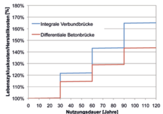
1 Kostenvergleich: Rahmenbrücke in Verbundbauweise und Zweifeld-Betonbrücke © Aus [2] [3]
