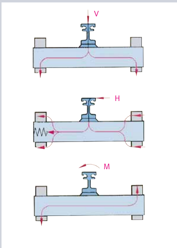
Lastabtragung am Mittelträger
