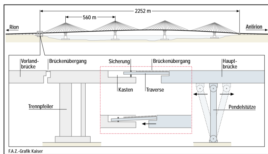
Bei einem schweren Erdbeben versagen die an beiden Enden des 2252 Meter langen Fahrbahntrags sitzenden Brückenübergänge kontrolliert: Sie rutschen unter die Fahrbahn in einen Kasten. Dabei werden sie zwar beschädigt, können aber von langsam fahrenden Rettungsfahrzeugen weiter benutzt werden. (kff)
